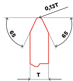
M MOLA A DISCO PROFILATA
