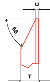
U MOLA A DISCO PROFILATA
