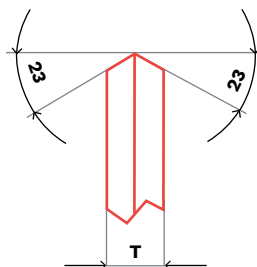
K MOLA A DISCO PROFILATA
