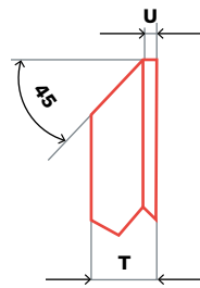
C MOLA A DISCO PROFILATA
