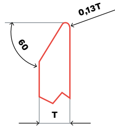
D MOLA A DISCO PROFILATA
