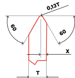
P MOLA A DISCO PROFILATA
