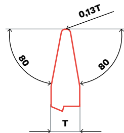
N MOLA A DISCO PROFILATA
