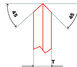
P MOLA A DISCO PROFILATA
