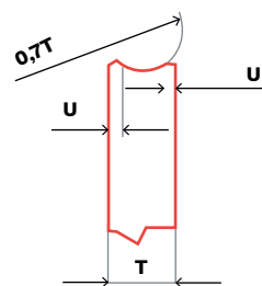
J MOLA A DISCO PROFILATA
