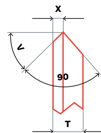
N MOLA A DISCO PROFILATA
